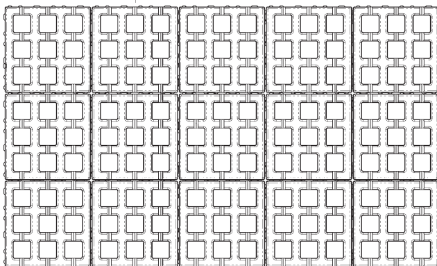
Quadro Radial Rasenstein 25 x 25 cm Abmessung ca. 125 x 75 cm, 15 Steine pro Lage
