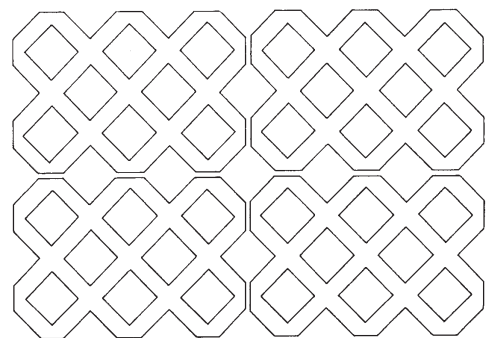
Rasengitter Abmessung ca. 120 x 80 cm, 4 Steine pro Lage
