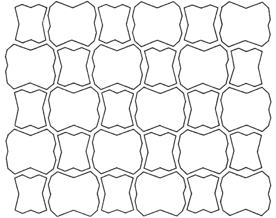
SUPRA® Radial-Öko Abmessung ca. 131 x 99 cm, 30 Steine pro Lage
