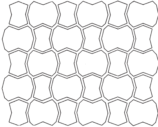
SUPRA® Radial Abmessung ca. 131 x 99 cm, 30 Steine pro Lage
